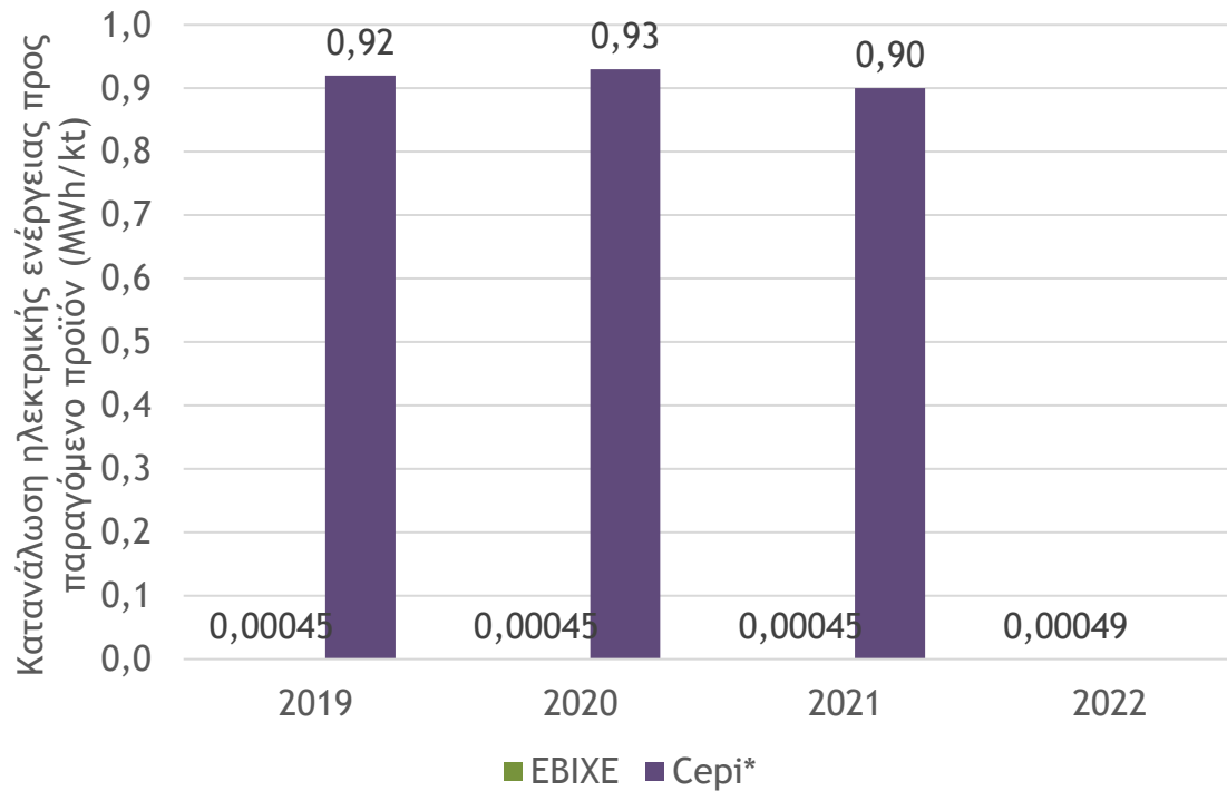
Δείκτης Έντασης Κατανάλωσης Ηλεκτρικής ενέργειας
