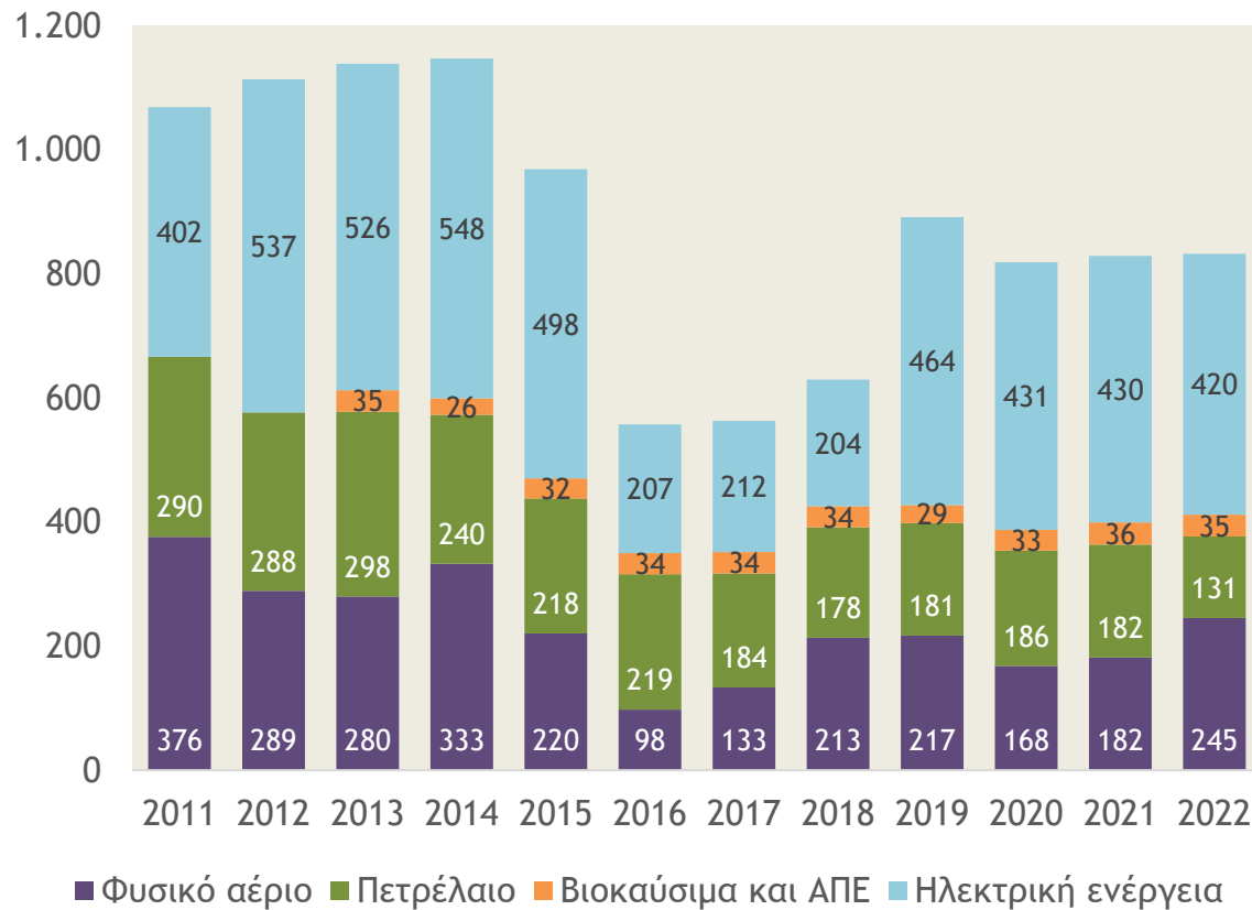
Τελική κατανάλωση ενέργειας ανά πηγή ενέργειας στη Βιομηχανία Χάρτου
